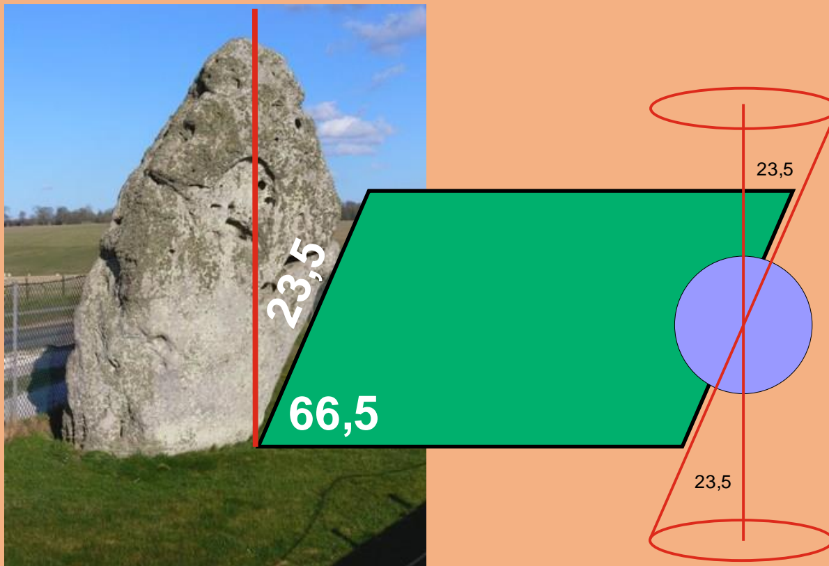
Aarde met precessiehoek
